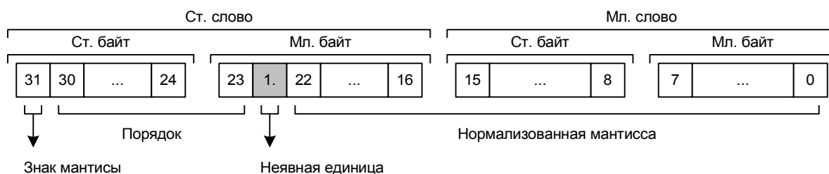
Рис. 3.1. - Формат FLOAT.
