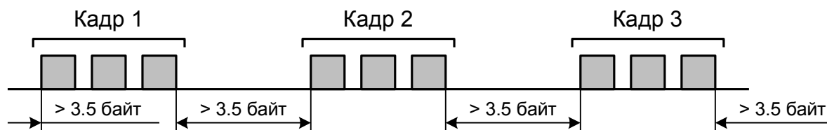
Рис. 2.4. – Пример передачи последовательности кадров.
